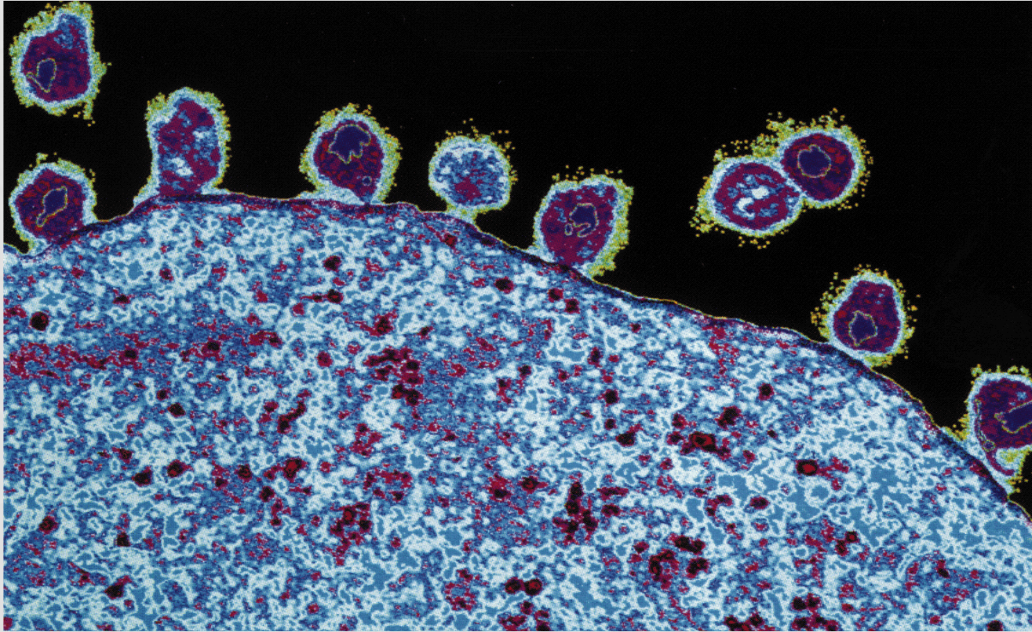
Электронная микрофотография вируса, выделяющегося из CD4 клетки
